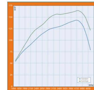
MOTORKENNLINIE Leistung normal: max. 103 kW (140 PS) Leistung mit Autologic: max. 119 kW (162 PS) Max. Leistungszunahme: 22 kW (30 PS) bei 3250 U/min
